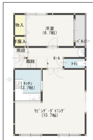
〈2階平面図〉
